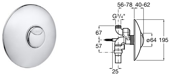
Fluxores para inodoros AQUA FLUXOR EMPOTRABLE DE 3/4". DOBLE DESCARGA 6/3 LITROS CON ROSETON. TUBO RECTO PARA INODORO. TECNOLOGÍA TEMPORIZADA. CROMADO .
