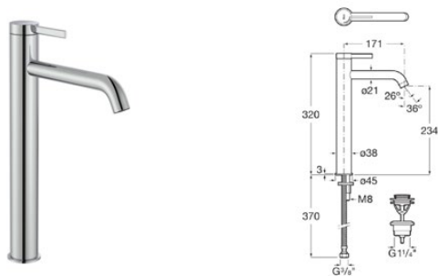
Ona MEZCLADOR MONOMANDO
