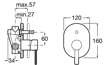
Mezclador empotrable A5A0 609 C00 $ 4,190.00
