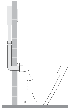
Con fluxor de empotrar 5A9 779 C00
