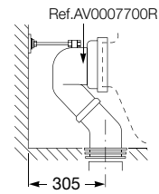
Con fluxor exterior 506 902 110
