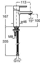
Mezclador monomando A5A3 296 C00 $ 1,980.00
