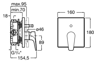
Mezclador empotrable A5A0 B90 C00 $ 2,900.00
