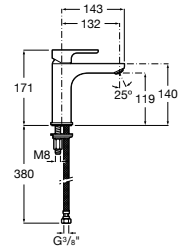
Mezclador monomando A5A3 B09 C00 $ 2,630.00
