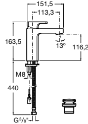
Mezclador monomando A5A3 901 C00 $ 6,420.00
