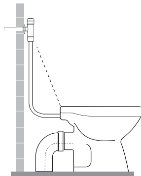
Con fluxor exterior 506 902 110
