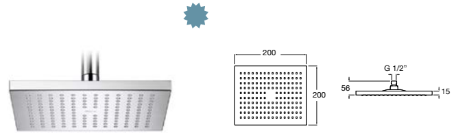
Rainsense rociador A5B2 350 C00 $ 2,470.00
