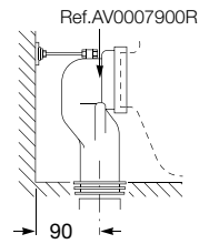
Con fluxor de empotrar 5A9 779 C00
