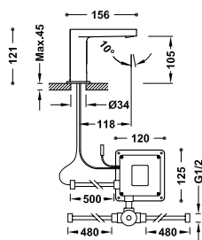
Grifo electrónico con sistema premezclador para lavabo Accionado mediante sensor de infrarrojos. Incluye una válvula mezcladora de 2 aguas con tubos flexibles (ref.: 19250730).
