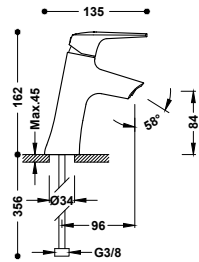
Grifo monomando inclinado para lavabo Latiguillos de alimentación flexibles G3/8.
