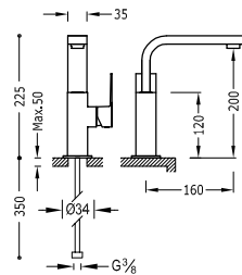
Grifo monomando con maneta lateral para lavabo Latiguillos de alimentación flexibles G3/8.
