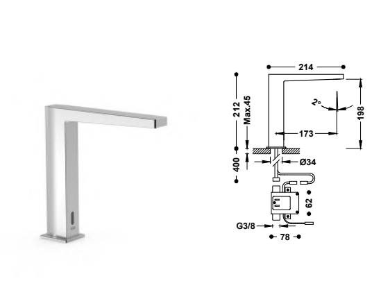
Grifo electrónico de 1 agua para lavabo Accionado mediante sensor de infrarrojos.
