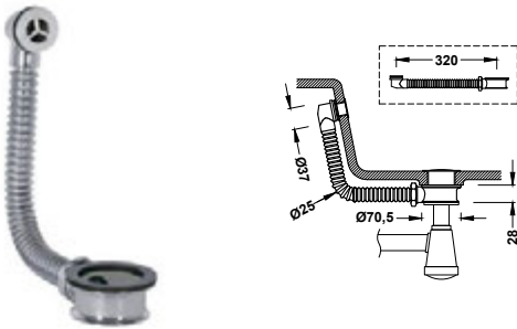
Adaptador para lavamanos de cristal o acero inoxidable que no poseen rebosadero Con rebosadero. Tubo flexible: 320 mm.
