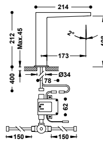
Grifo electrónico con sistema premezclador para lavabo Accionado mediante sensor de infrarrojos. Incluye una válvula mezcladora de 2 aguas con tubos flexibles (ref.: 19250730).
