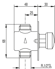
Grifo de descarga temporizado empotrado de 1 agua para urinario
