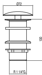
Válvula de desagüe siempre abierto para lavabo sin rebosadero Sin rebosadero. Tapón: Ø 72 mm.
