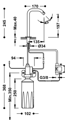
Grifo electrónico de 1 agua con dispensador de jabón automático para lavabo Accionado mediante sensor de infrarrojos. Capacidad del depósito de jabón: 1600 ml.
