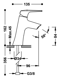
Grifo monomando inclinado ecoeficiente para lavabo Latiguillos de alimentación flexibles G3/8.
