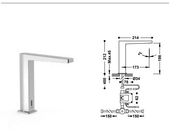
Grifo electrónico con sistema premezclador para lavabo Accionado mediante sensor de infrarrojos. Incluye una válvula mezcladora de 2 aguas con tubos flexibles (ref. 19250730).
