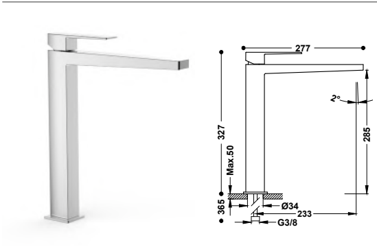
Grifo monomando XXL para lavabo Latiguillos de alimentación flexibles G3/8.
