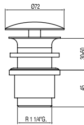
Válvula de desagüe siempre abierto para lavabo sin rebosadero Sin rebosadero. Tapón: Ø 72 mm.
