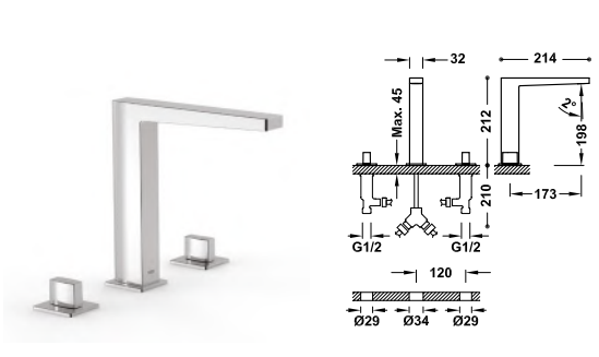
Grifo bimando de repisa para lavabo De instalación libre. Con volantes.
