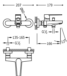
Grifo monomando mural para bañera y ducha Ducha de mano anticalcárea. Soporte orientable para ducha de mano. Flexo satinado.
