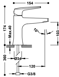
Grifo monomando ecoeficiente para lavabo Latiguillos de alimentación flexibles G3/8.
