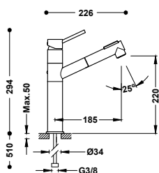
Grifo monomando con caño extraíble con 2 tipos de chorro para cocina Con latiguillos de alimentación flexibles G3/8.
