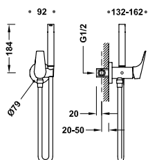
Grifo monomando empotrado con ducha para inodoro Con agua fría o caliente. Ducha de mano con racor limitador a 5 l/min. y sistema antigoteo. Soporte fijo para la ducha de mano instalable a derecha o izquierda. Flexo satinado.
