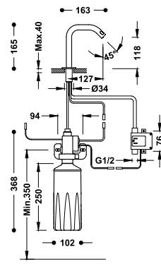
Grifo electrónico de 1 agua con dispensador de jabón automático para lavabo Accionado mediante sensor de infrarrojos. Capacidad del depósito de jabón: 1600 ml.
